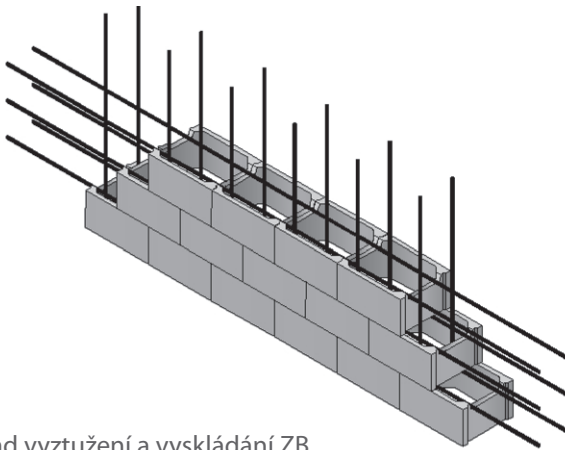
Příklad vyztužení a vyskládání ZB
